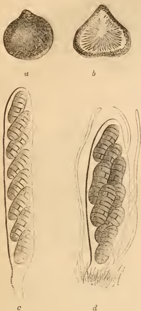
Fig. 68. Sphaeria herbarum .
