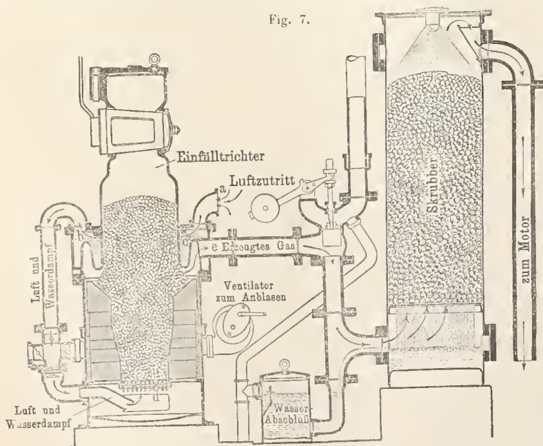
Schema einer Sauggasgenerator-Anlage.
