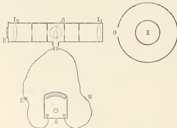
Ein Körper K , dessen Temperatur bestimmt werden soll, befindet sich in einem Ofen mit der Öff-
