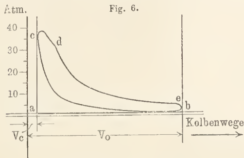
Indikatordiagramm des Dieselmotors.
