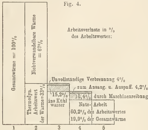
Arbeitsbilanz des 10 PS. Göttinger Leuchtgasmotors.
