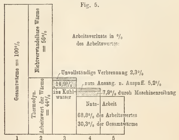
Arbeitsbilanz einer 70 PS. Braunkohlengasmaschine.
