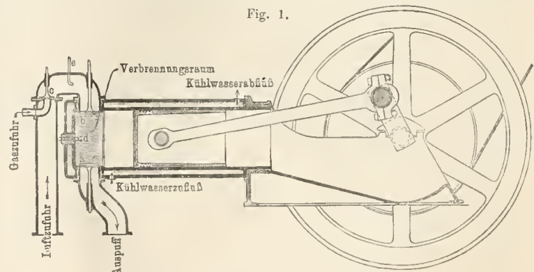
Schematischer Längsschnitt einer Gasmaschine.
