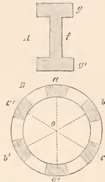
Fig. 55. A ein I-förmiger Träger, g obere, g' untere Gurtung, f Füllung des Trägers. B zusammengesetzter Träger, aus drei I-förmigen kombiniert; a, a' , b, b' , c, c' die drei Gurtungspaare; durch o geht die gemeinschaftliche neutrale Achse.
