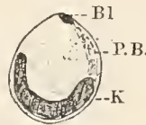
Chr Chromosomen, Bl Blepharoplast, K Kern, P. B. Plasmaband, Z. P. Zentrales Plasma (Vorderende des Spermatozoids).
