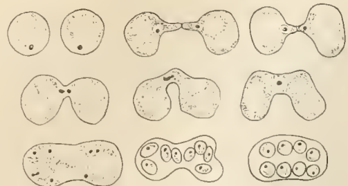
Schizosaccharomyces octosporus . Kopulation und Ascusbildung. Nach Guilliermond.
