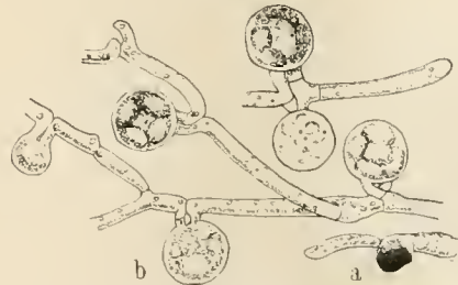
Eremascus fertilis . Bei a die Sporenmembran mit dem keimenden Mycel. Nach Rose Stoppel.
