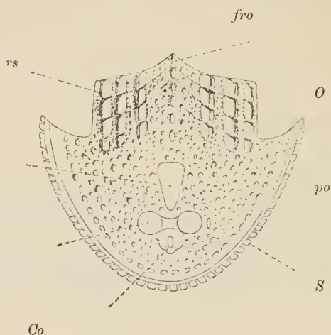
Figur 4. Thyestes verrucosus , EICHWALD. Obersilar von der Insel Oesel in Russland Oberes Kopfschild. 28) O = Augenöffnungen, fro = Frontalorgan, po = Parietalorgan, S = segmentartige Hautplatte, Co = Crista occipitalis , rs = Randhöcker Zweimal vergrößert.
