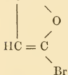
Bromfurfurdibrompropionic Acid.
