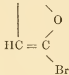
Bromfurfurethylen.
