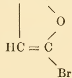
Bromfurfuracrylic Acid.
