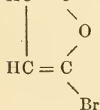
Bromfurfurbromacrylic Acid.
