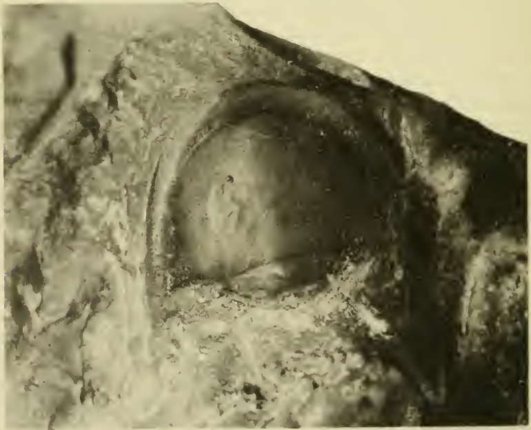
Fig. 17. Typhloproetus microdiscus Frech, blinder Trilobit aus dem obersten Devon der Karnischen Alpen, 13 : 1 nat. Gr.
