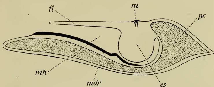
Fig. 31. Cymbalia peroni Blainville. Schematischer Durchschnitt, senkrecht zur Fläche der Figur 30, nach Meisenheimer.
