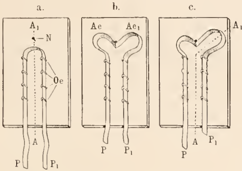
Fig. 4. Papierstreifenmodell zur Veranschaulichung des Auseinanderweichens zweier Zweigäste ( Ac , Ae_1 ).
