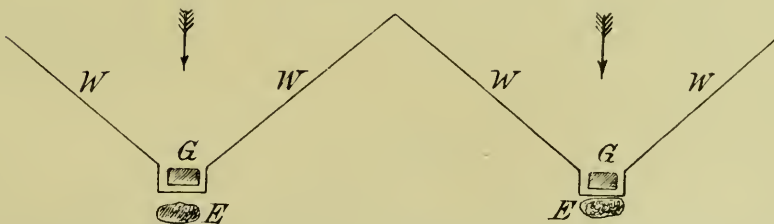
Fig. 132. Schema eines cyprischen Apparates (appareil Durand) (nach GUÉNAUX). W Wände, G Gräben, E Erdhaufen.
