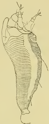
Fig. 13. Phyllocoptes ritis Nal., femmina, di fianco. Ingr. 375.
