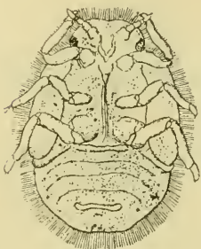
Fig. 31. Psyllide aus Blattgruben auf Stephania abyssinica ; 10: 1.
