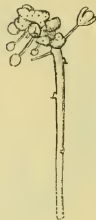
Fig. 147. Blütenstand- galle von Tinospora crispa Diels. \times 1 .
