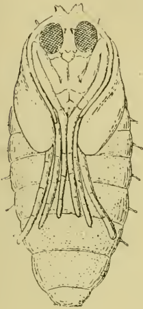
Fig. 4. Cecidomyidenpuppe aus Gallen auf Aca- lypha spec.; 21: 1.
