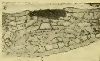
Fig. 3. Sezione di foglia di 420 A, con puntura di Phyllocoptes sulla pagina superiore (Noto). Ingr. 160.
