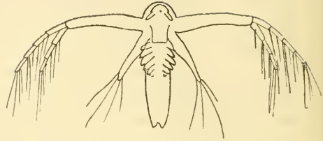
Fig. 2. Winterci— Metanauplius von Leptodora .
