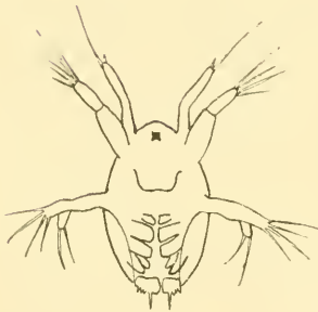
Fig. 5. Metanauplius von Euphausia .
