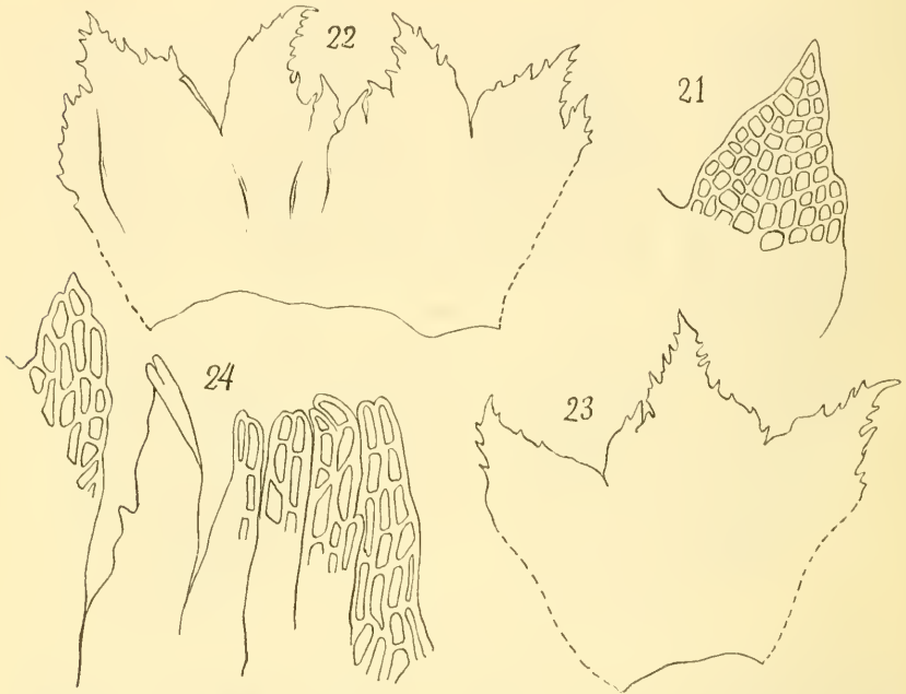
Cephaloziella Latzeliana f. Stanensis (von Slano, Nr. 221 b ). — Fig. 21. Teil eines Stengelblattes, Verg. 260 : 1. — Fig. 22, 23. Teile des Involucrum, Verg. 80 : 1. — Fig. 24. Teil der Perianthmündung, Verg. 260 : 1.
