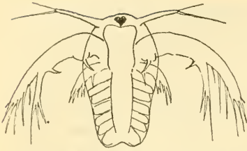
Fig. 1. Metanauplius von Apus .
