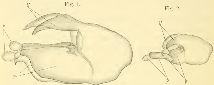
Fig. 1. Kopulationsapparat des ♂ von Lythria purpuraria L. (Penis entfernt.)
