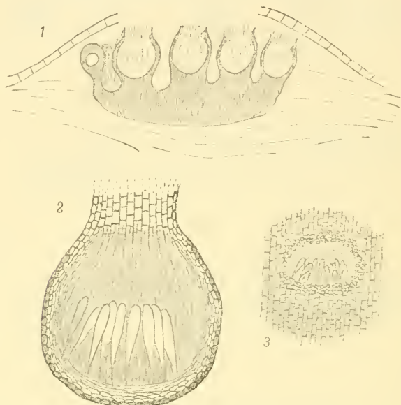
Fig. 4. 1 Botryosphaeria Dasylirii (Peck) Theiss. et Syd., Querschnitt; 2 Botryosphaeria Castaneae (Schw.) Sacc., ein Gehäuse im Querschnitt; 3 Botryosphaeria ventricosa (Mont.), ein Perithezium im Stroma. Alles nach den Originalen.
