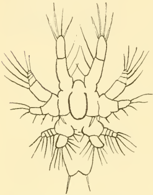
Fig. 3. Nauplius von Diaptomus .
