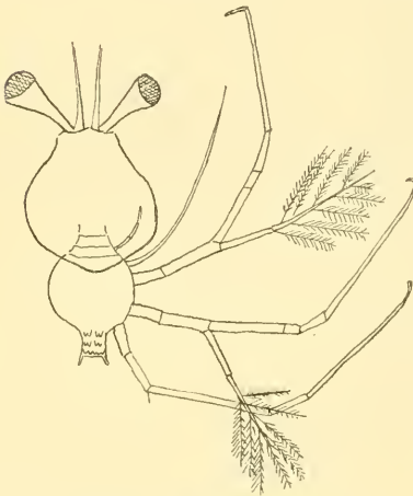
Fig. 15. Mysis -Stadium („Phyllosoma“) von Scyllarus .
