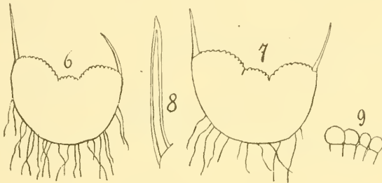
Riccia Crozalsi Lev. (von Ins. Giuppana, Nr. 245). — Fig. 6, 7. Querschnitte, Verg. 30:1. — Fig. 8. Randeilie, Verg. 87:1. — Fig. 9. Epidermiszellen, Verg. 87:1.
