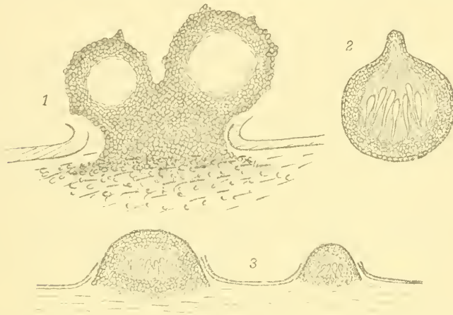
Fig. 6. 1 Botryosphaeria Bakeriana Rehm, Querschnitt; 2 Botryosphaeria acerina Rehm; 3 Botryosphaeria diplodioidea (D. et M.) Sacc. Alles nach den Originalexemplaren.
