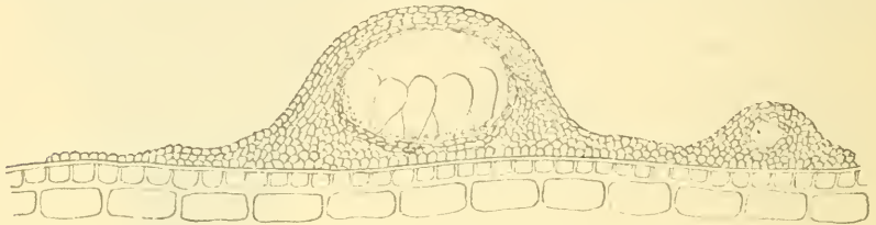
Fig. 2. Saccardinula guaranitica Speg. Querschnitt.
