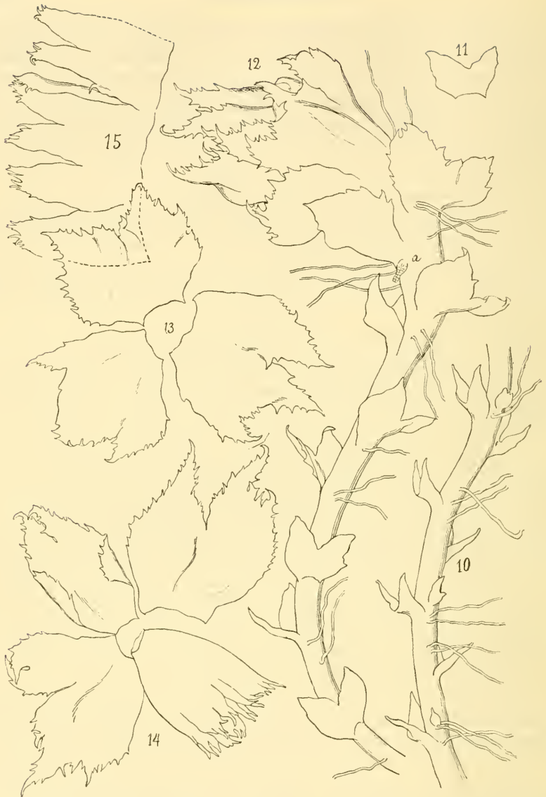
Cephaloziella Latzeliana Schffn. n. sp. (von Ins. Gnippana). — Fig. 10. Teil des sterilen Stengels. — Fig. 11. Blatt desselben. — Fig. 12. Pflanze mit Involucrum (bei a ein extraflorales Archegonium). — Fig. 13. Cyclois der Subinvolucralblätter. — Fig. 14. Involucrum und junges Perianth. — Fig. 15. Junges Perianth ausgebreitet. Alle Figuren verg. 60 : 1.
