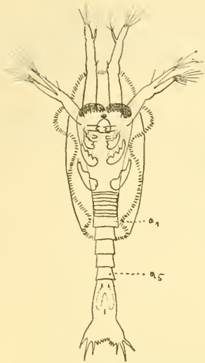
Fig. 7. Calyptopis (= Zoëa ) von Euphausia .
