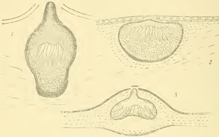
Fig. 1. 1 Pyreniella rhodina (B. et C.) Theiss.; Gehäuse im Querschnitt. 2 Cryptosporina abietina (Prill. et Delacr.) Theiss.; Fruchtkörper im Querschnitt. 3. Amerostegē pseudopustula (Br. et Har.) Theiss.; Querschnitt durch ein Stroma.
