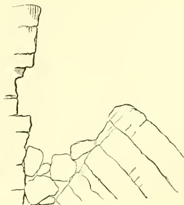
Fig. 28. Section of Cliff at Kalapànu.
