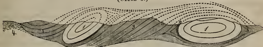
1. Bělokamen. 2. hadec. 3. rula. 4. žžula.
