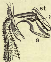
2647. Cypripedium .— st , staminodium; a , anther; s , stigma.
