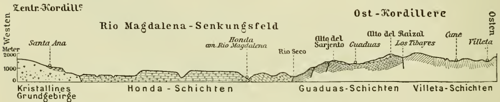
Profil durch das Magdalenatal und seine Randgebiete bei Honda. (Nach H. Stille.) Zu S. 407.
