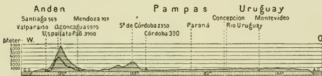
Querschnitt über Südamerika unter 33° südl. Breite, 50fache Überhöhung. Zu S. 52.
