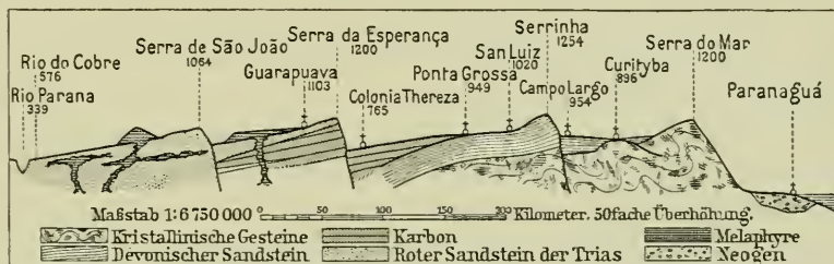
Quersprofil über Südbrasilien unter 26° süd. Breite. (Nach J. v. Siemiradzki.)
