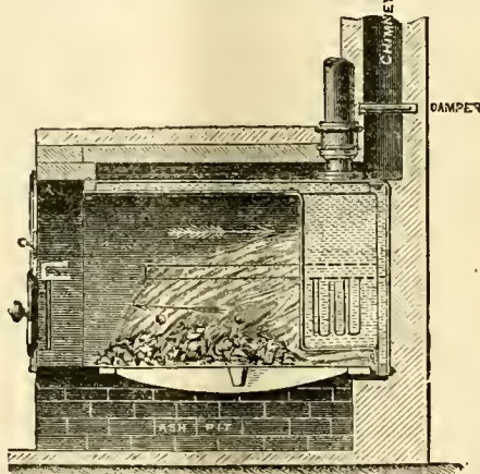
— LONGITUDINAL SECTION —
