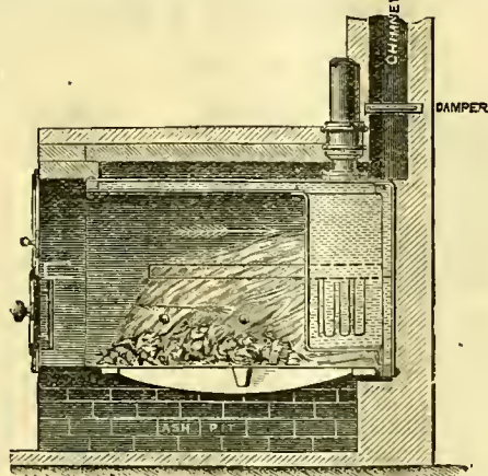
— LONGITUDINAL SECTION —
