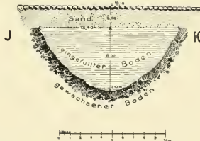
Fig. 5. Plan und Schnitte der Grabungen in der Mönckebergstraße: Spuren der Stadtbefestigung des 12. Jahrhunderts. (Nach Aufnahmen der Direktion der Gaswerke)
