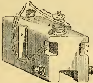
("CLIMAX" BOILER.)
