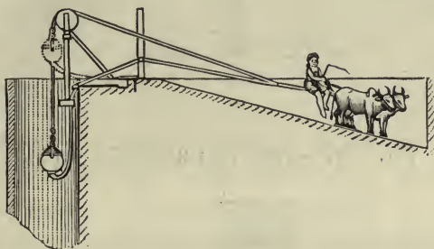
FIG. 36.—THE SINGLE MÔT.
