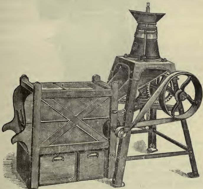
FIG. 54.—BALMER & LAWRIE'S PADDY-HUSKER.
