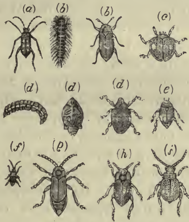
FIG. 66.—COLEOPTERA.
