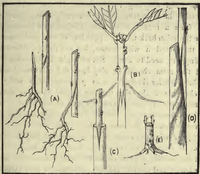
FIG. 59.—GRAFTING.
