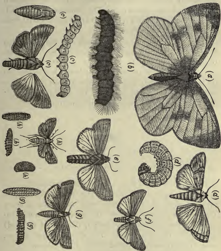
FIG. 67.—LEPIDOPTERA.
