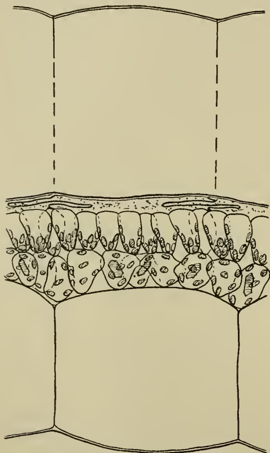
Fig. 2. Blattquerschnitt durch den abgeschliffenen Teil von Beg. semperflorans nach Beendigung des vollständigen Versuches. Das Material stammt vom Versuch 1 (S. 497). Die ursprüngliche Form der oberen Epidermis ist punktiert eingetragen (gezeichnet nach Präparaten durch den intakten Teil desselben Blattes).
