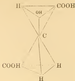
l-Apfelsäure:
