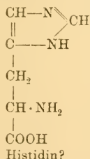
Histidin?
