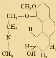
Codein
