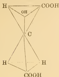
Crassulaceenapfelsäure:
