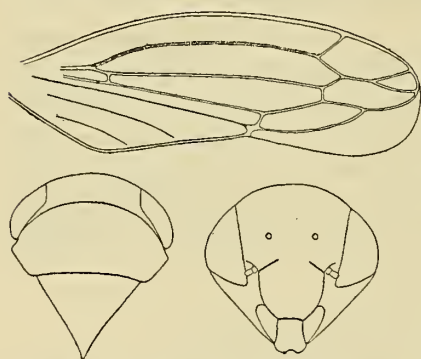
FIG. 23. Idiocerinus nacreatus sp. nov.
