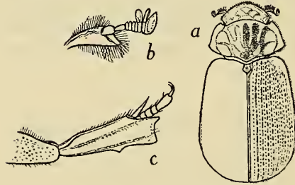
FIG. 2. a, Trox montalbanensis sp. nov.; b, linke Antenna von unten; c, linkes Vorderbein von unten.
