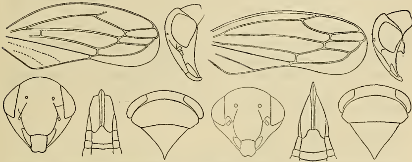
FIG. 13. Pedioscopus modestus sp. nov.
