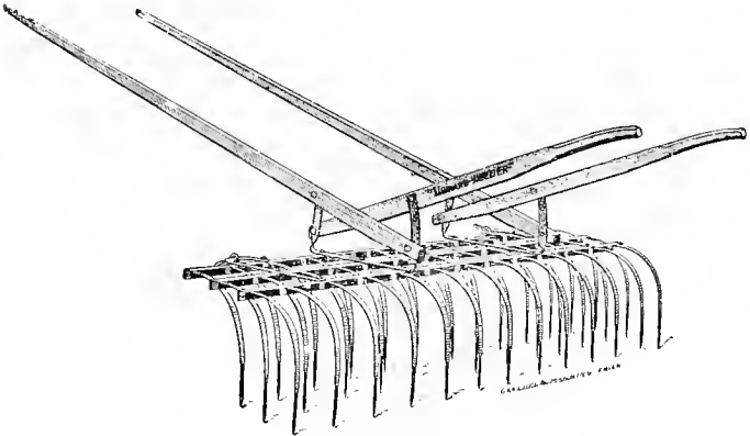
FIG. 86. — A WEEDER.
