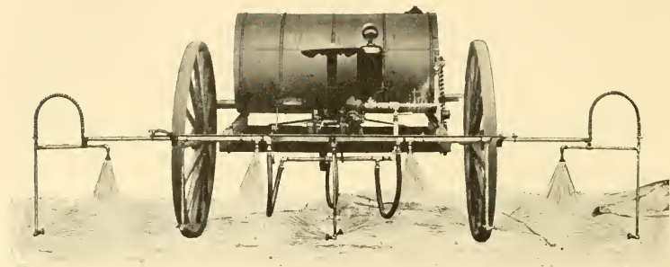
Abb. 113. Fahrbare Kartoffelspritze. Nach Appel.
