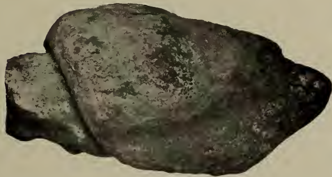
Figs. 1-3. Voluta sp. indet.
