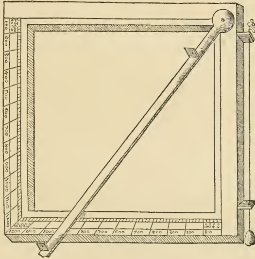
Abb. 59. Peurbachs Quadratum geometricum 3) .
