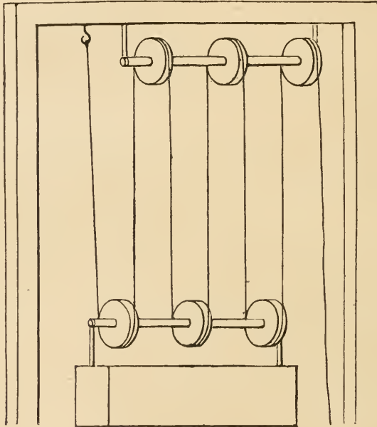
Abb. 33. Herons Flaschenzug.
