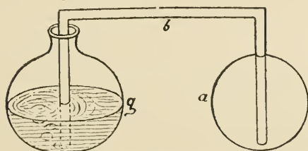
Abb. 31. Philons Thermoskop.
