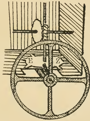
Abb. 34. Herons Wegmesser 3) .
