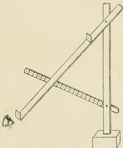
Abb. 45. Das parallaktische Lineal.
