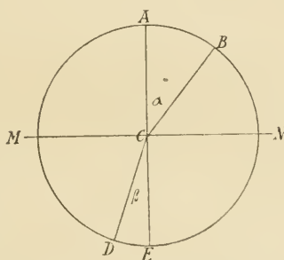
Abb. 47. Ptolemäos mißt die Brechungswinkel.
