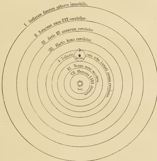
Abb. 62. Das kopernikanische Weltsystem.
