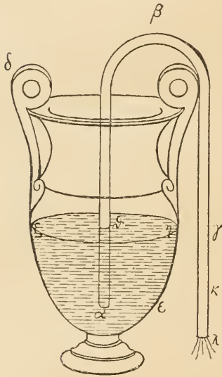
Abb. 28. Herons Abbildung eines Hebers.
