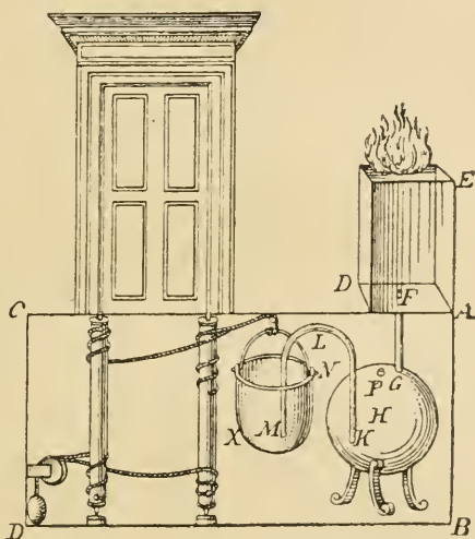
Abb. 29. Herons Automat zum Öffnen der Tempeltür 1) .
