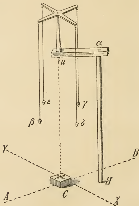
Abb. 39. Die Rekonstruktion der Groma.
