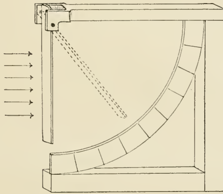
Abb. 57. Lionardos Windmesser.
