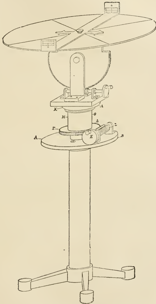
Abb. 35. Herons Winkelmeßapparat.
