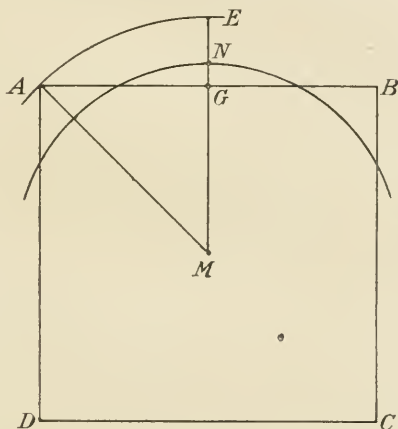
Abb. 10. Die Quadratur des Kreises bei den Indern.
