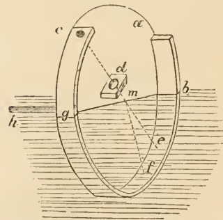
Abb. 54. Alhazen untersucht die Brechung.
