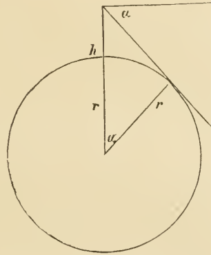
Abb. 50. Albirunis Bestimmung des Erdumfanges.
