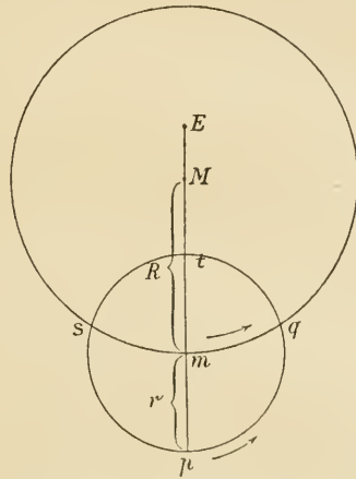
Abb. 44. Zur Erläuterung der Epizyklentheorie.
