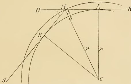
Abb. 55. Alhazen bestimmt die Höhe der Atmosphäre.
