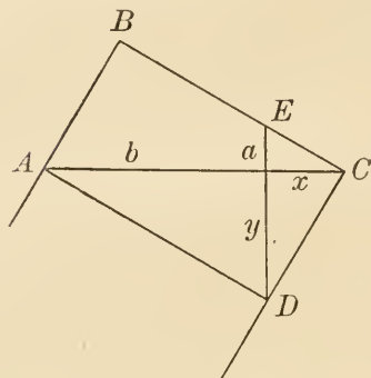
Abb. 13. Konstruktion zur Lösung des delischen Problems.
