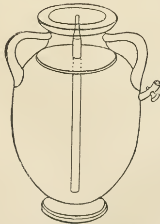
Abb. 27. Der Heronsball.
