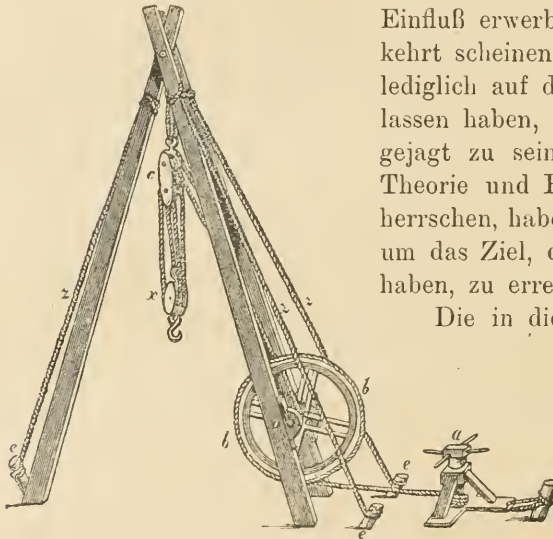
Abb. 41. Römisches Hebezeug 2 .
