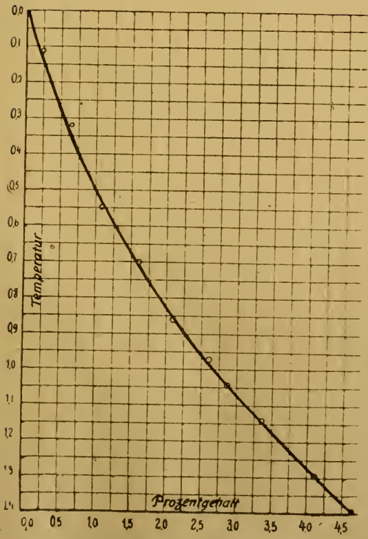
Kurventafel 10 (zu Tabelle 21).
