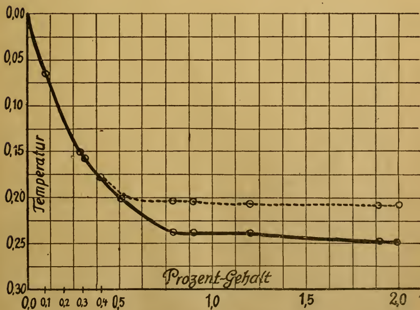
Kurventafel 2 (zu Tabelle 9).
