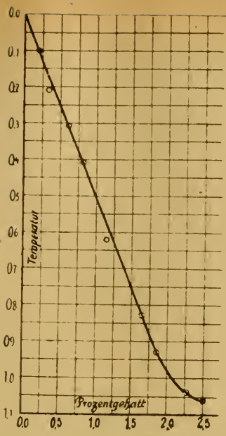
(Kurventafel 9 zu Tabelle 20).
