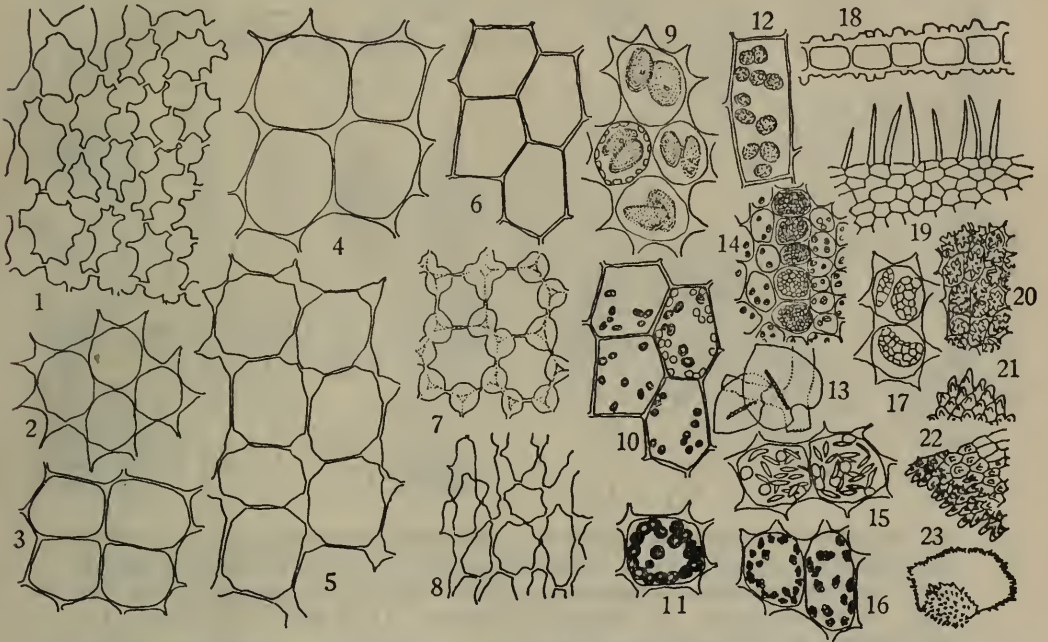
图 8 苔类植物叶细胞及油体形状 1—8.苔类的细胞形状和细胞壁加厚示例: 1. 毛叶苔叶片的细胞, 2. 钱袋苔叶片的细胞, 3—7. 合叶苔属代表类型的叶细胞, 8. 耳叶苔叶片的细胞; 9—17. 苔类细胞中的油体形状: 9. 钱袋苔叶片细胞中的油体, 10. 合叶苔叶片细胞中的油体, 11、12. 裂叶苔属叶片细胞中的油体, 13、14. 耳叶苔叶片细胞中的油体, 15. 鳃叶苔叶片中的油体, 16. 瘤萼苔叶片中的油体, 17. 唇鳞苔属叶片细胞中的油体(东北地区无此种), 18—23. 苔类细胞壁疣突示例: 18. 合叶苔属的少数种, 19. 叉苔属的毛状突起, 20. 疣鳞苔属的星形疣(东北地区无此种), 21—23. 疣鳞苔属的单锐疣(东北地区无此种)。
