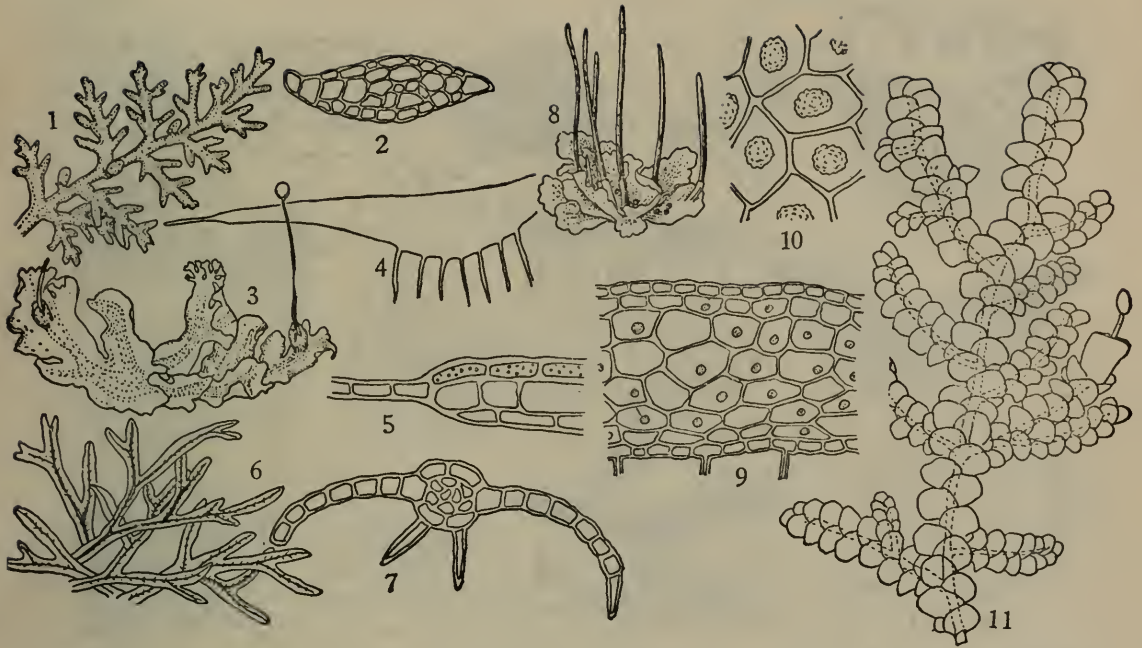
图2 苔类植物体及其构造 1—2. 片叶苔属 ( Riccardia ): 1. 植物体, 2. 植物体的横切面; 3—5. 溪苔属 ( Pellia ): 3. 植物体, 4. 植物体的横切面, 5. 植物体横切面近边的一部分; 6—7. 叉苔属 ( Metzgeria ): 6. 植物体, 7. 植物体的横切面; 8—9. 角苔属 ( Anthoceros ): 8. 植物体, 9. 植物体横切面的一部分, 10. 叶状体细胞放大, 11. 扁萼苔属 ( Radula ) 植物体。
