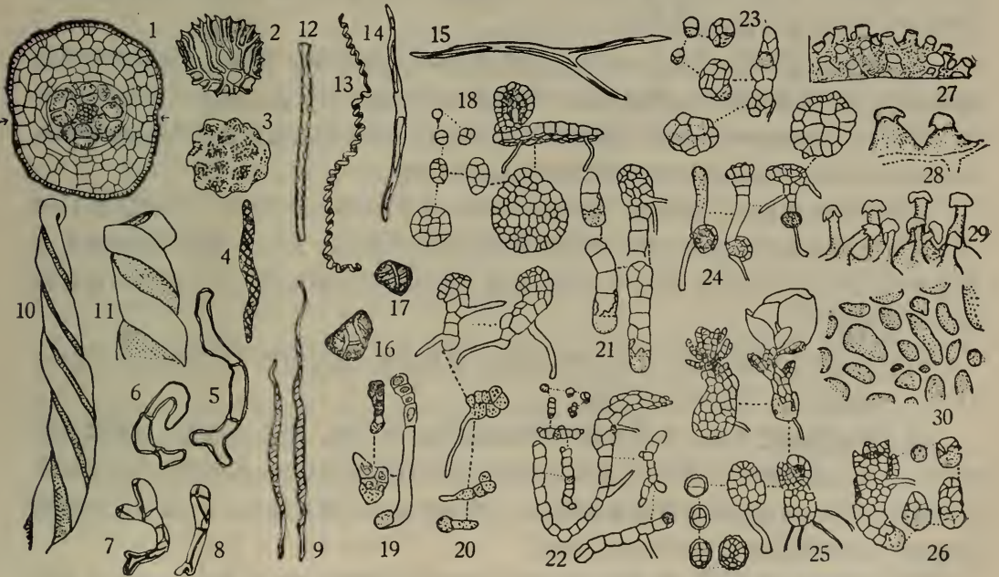
图 13 苔类植物的孢子、弹丝及孢子萌发后的原丝体 1. 角苔孢蒴的横切面, 2. 小叶苔孢子, 3. 皮叶苔孢子, 4. 钱袋苔的弹丝, 5—8 角苔属的假弹丝, 9. 叉苔属的假弹丝, 10、11. 两条螺纹的弹丝一端放大, 12. 鳞苔属的弹丝, 13. 光萼苔属的弹丝, 14, 15. 无纹紫背苔分化不完全的弹丝, 16、17. 短角苔的假弹丝, 18. 扁萼苔属的孢子萌发和原丝体, 19. 角苔属的孢子萌发和原丝体, 20. 地钱的孢子萌发和原丝体, 21, 26. 合叶苔属的孢子萌发和原丝体, 22. 大萼苔孢子萌发和原丝体, 23. 被蒴苔属的孢子萌发和原丝体, 24. 石地钱的孢子萌发和原丝体, 25. 耳叶苔的孢子萌发和原丝体, 27. 剪叶苔孢子表面疣, 28. 复叉苔孢子的表面疣, 29. 光萼苔孢子的表面疣, 30. 皮叶苔孢子表面的小凹。(部分仿 M. Schuster)。
