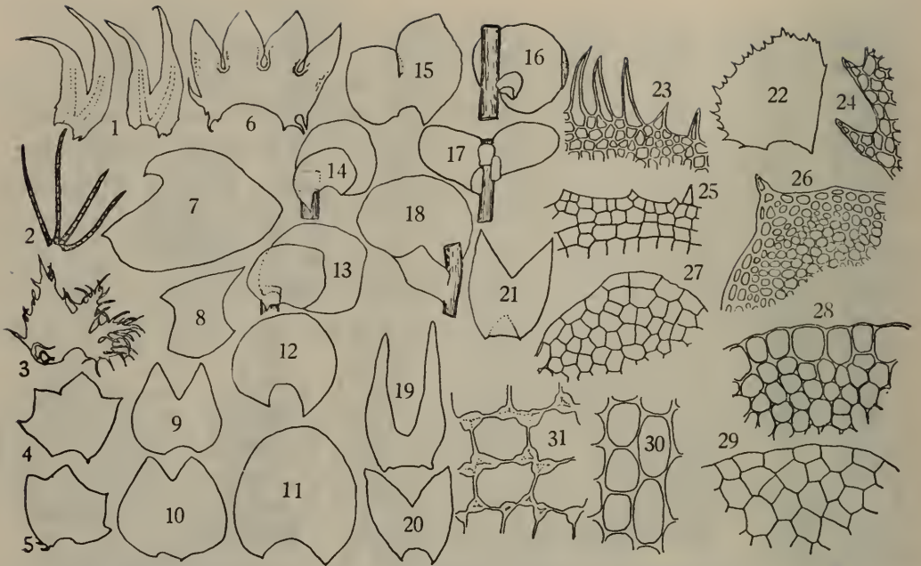
图7 苔类植物的叶片形状及叶缘 1—22. 苔类的叶片形状示例: 1. 剪叶苔2裂叶片, 2. 睫毛苔裂成毛状的叶片, 3. 毛叶苔叶片, 4—6. 裂叶苔的叶片形状, 7. 护蒴苔叶片, 8. 裂叶苔二裂瓣叶片, 9、10. 钱袋苔二裂瓣叶片, 11. 12. 圆叶苔叶片, 13—15. 合叶苔背瓣小腹瓣大叶片, 16. 耳叶苔腹瓣特化成囊状的叶片, 17. 光萼苔背瓣大腹瓣小的叶片, 18. 扁萼苔叶片, 19. 大萼苔二裂的叶片, 20. 拟大萼二裂叶片, 21. 兔耳苔二裂叶片, 22、23、25、26. 合叶苔代表种的叶缘, 24. 羽苔的叶缘具多细胞齿, 27、29. 护蒴苔属的叶缘, 28. 贝萼苔属的部分种叶缘细胞, 30、31. 剪叶苔的叶细胞。
