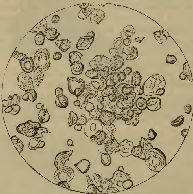
Fig. 466. — Grains de fécule de tapioca altérés par la chaleur employée pendant la préparation (grossissement de 225 diamètres). (Hassall).
