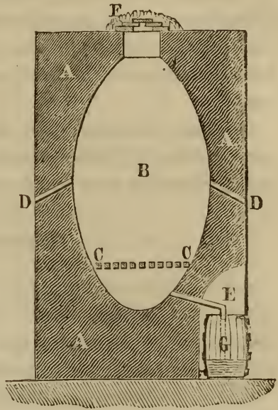
Fig. 423. — Four à préparer le goudron (*).
