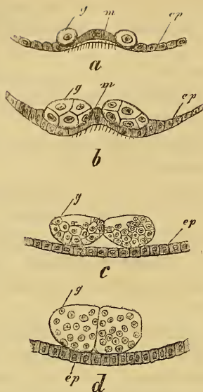
Obr. II. Znázornění vývoje ganglia u annulátů a členovců.
