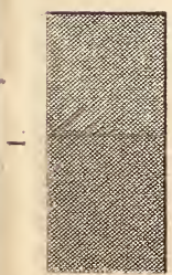
Roches rhyolites.
