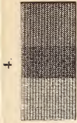
Roches métamorphiques.
