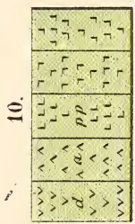
Dichastites.
