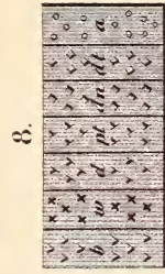
Basaltites.
