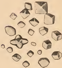
Fig. 27. Kristalle von Ammonium- phosphormolybdat. Vergr. 350.
