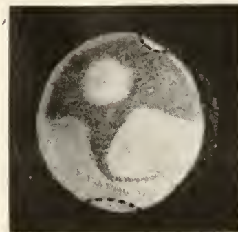
Fig. 4. Mars am 10. April 1895. (Durchmesser: 5'')
