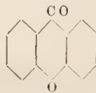
Xanthon.
