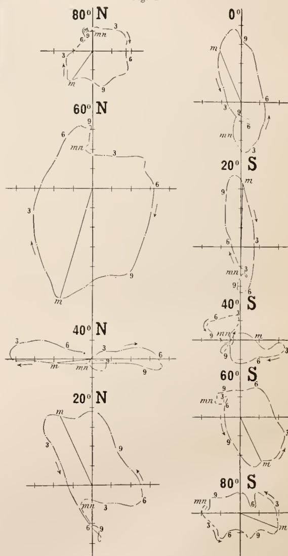
Vectordiagramme der täglichen Variation des Erdmagnetismus für das Sommerhalbjahr der nördlichen Halbkugel.
