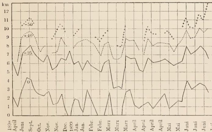
Diagramm der Höhen, in welchen man zu verschiedenen Zeiten die Isothermen von 0°, -25°, -40°, -50° angetroffen. Die Isothermen -40° und -50° fehlen bei einigen Aufstiegen, da die Ballons nicht hoch genug gestiegen waren, um sie zu treffen.
