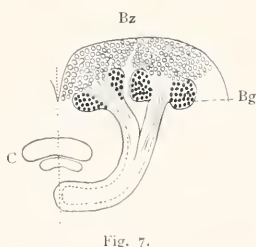
Fig. 3—8. Schemata der pilzförmigen Körper und des Zentralkörpers C im Gehirn von: Fig. 3 Tomocerus flavescens (Springschwanz (nach Kühnle), Fig. 4 Silberfischchen (nach Böttger), Fig. 5 Lederlaufkäfer, Fig. 6 Mehlkäfer, Fig. 7 Goldkäfer, Fig. 8 Küchenschabe. Bei Fig. 5 und 7 sind die rückläufigen Stiele weggelassen. Bz Becherzellen; Bg Becherglomerulen; P Plzstiele; R rückläufiger Stiel; Ba Balken; Tn Trauben. Die punktierte Linie ist die Medianlinie (Symmetrieebene).
