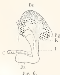
Fig. 3—8. Schemata der pilzförmigen Körper und des Zentralkörpers C im Gehirn von: Fig. 3 Tomocerus flavescens (Springschwanz (nach Kühnle), Fig. 4 Silberfischchen (nach Böttger), Fig. 5 Lederlaufkäfer, Fig. 6 Mehlkäfer, Fig. 7 Goldkäfer, Fig. 8 Küchenschabe. Bei Fig. 5 und 7 sind die rückläufigen Stiele weggelassen. Bz Becherzellen; Bg Becherglomerulen; P Plzstiele; R rückläufiger Stiel; Ba Balken; Tn Trauben. Die punktierte Linie ist die Medianlinie (Symmetrieebene).
