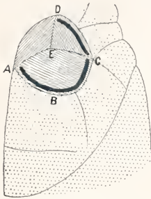
Schema eines Stückes der Felsoberfläche, aus dem der Teil A—E durch Hammerschlag entfernt ist, um die Endolithenbänder zu zeigen.
