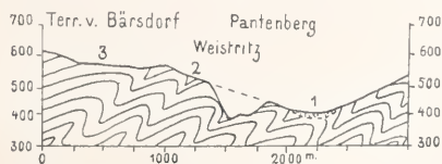
Abb. 1. Rezentes und mit Geschiebelehm erfülltes diluviales Tal der Weistritz. (Maßstab 1:50000, 2\frac{1}{2} mal überhöht.)
