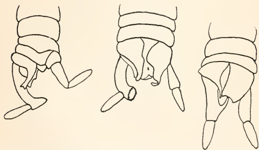
Fig. 9. Hinterleibsende männlicher Embien (von oben) nach Krauß. (Behaarung weggelassen.)
