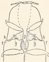
Fig. 2. Vorderer Teil eines Schnellkäfers ( Athous rufus Degeer), von unten gesehen. D Dorn, G Grube, v Vorsprung am Hinterrand des Prostrernum, h hinterer seitlicher Vorsprung des Hinterrandes des Prostrernum, f Gelenkfurchen zur Aufnahme des Vorsprunges h. Vergr. 5 : 1. (Nach Prochnow.)
