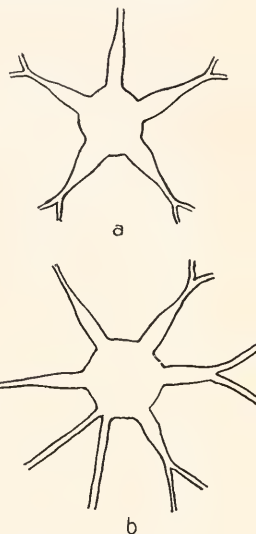
Fig. 13. Radiarkanäle von Cladonema radiatum . a) noch bilateral symmetrisch, b) ganz asymmetrisch.
