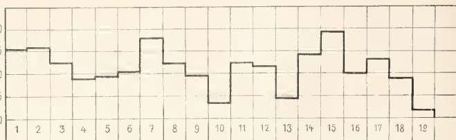
Abb. 7. Teilungsgeschwindigkeit von Stylonychia. Nach den Zahlen von Popoff. Durchschnittswerte für Perioden von fünf Tagen. (Nach Gregory, Aus Woodruff und Erdmann.)
