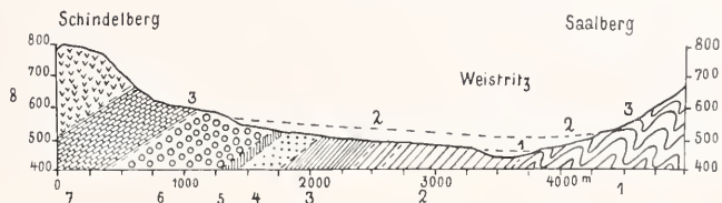
Abb. 3. Querprofil des oberen Weistriztales. (1 Gneis; 2 Sandsteine, 3 Konglomerate des Ob. Karbon (Waldenburger und Saarbrücker Sch.); Unteres Rotliegendes: 4 braunrote Sandsteine, 5 Schiefer, 6 Konglomerate der Unteren Kuseler Sch.; 7 Bausandsteine der Oberen Kuseler Sch.; 8 Quarzporphyr (mittl. Rotliegendes). Maßstab 1:50 000, 2 1/2 mal überhöht.
