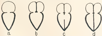
Fig. 1. Schemata der Kammern und Vorkammern des Herzens bei den Wirbeltieren.
