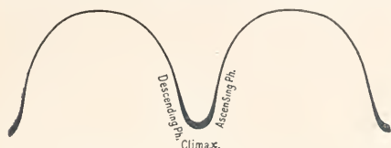
Abb. 3. Schematische Darstellung des Rhythmus (Nach Woodruff und Erdmann.)
