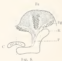
Fig. 3—8. Schemata der pilzförmigen Körper und des Zentralkörpers C im Gehirn von: Fig. 3 Tomocerus flavescens (Springschwanz (nach Kühnle), Fig. 4 Silberfischchen (nach Böttger), Fig. 5 Lederlaufkäfer, Fig. 6 Mehlkäfer, Fig. 7 Goldkäfer, Fig. 8 Küchenschabe. Bei Fig. 5 und 7 sind die rückläufigen Stiele weggelassen. Bz Becherzellen; Bg Becherglomerulen; P Plzstiele; R rückläufiger Stiel; Ba Balken; Tn Trauben. Die punktierte Linie ist die Medianlinie (Symmetrieebene).
