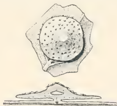
Fig. 2. Neuroterus lenticularis \frac{3}{4} (nach Roß). Darunter ein Längsschnitt, der die Larvenkammer zeigt.
