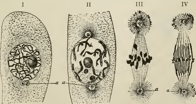
Fig. 5. Lilium Martagon . I. Spitze des Embryosackes. II. Id. älteres Stadium. III. und IV. Vorgeschrittene Kerntheilungsfiguren ebendaher. Zeigen die Theilung der Attractionssphären (a). Nach Guignard aus Zimmermann, Botanische Mikrotechnik, p. 193.
