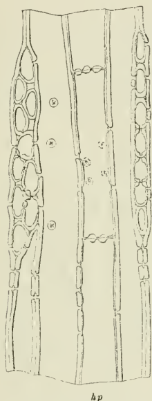
2. rajz. Thuja occidentalis egy- és kétszoros vastag bélsugarai. hp hosszparenchymsejtek. 300-szor nagyítva.
