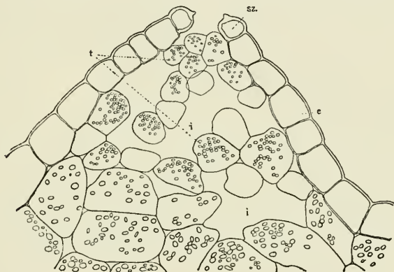
7. kép. Szárazon hajtattott gumó sarjain képződött fiatal lenticella km.-e. e) epidermis. — sz.) a csúcsi levegőnyílás zárósejtjei. — t) keményítő és klorofill tartalmú töltősejt; — i) sejtközök.
