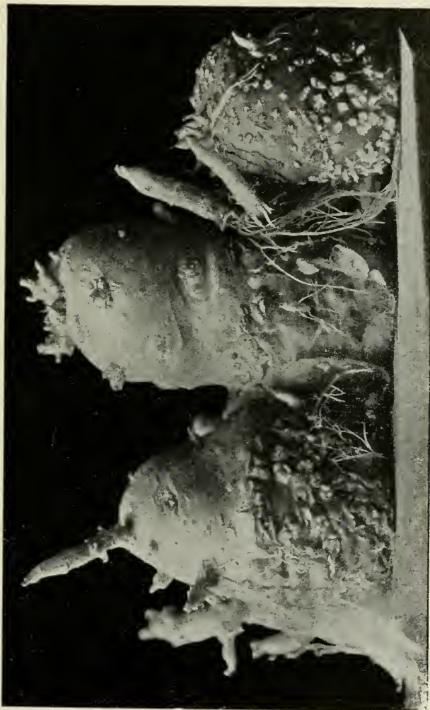
1. kép. A burgonyagumók kérgének aërenchimás burjánzása. Mind a három gumót fele magasságig vízbe állítva hajtattam. A balról számított I. és II. gumó felső fele hajtás alatt száraz levegővel érintkezett. A vizalatti részen az aërenchimás kinövések és a szabad felületen a megdagadt lenticellák láthatók. A III. gumó vízfeletti részét a hajtás alatt páratelt levegő vette körül és ennek következtében az aërenchimás kinövések az egész felületén megjelentek.
