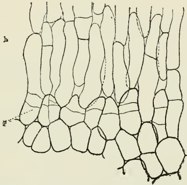
8. kép Peridermalépződés kezdete az aërenchimás zóna alatt. (Részlet a gumó hipertrofiás kérgének km.-éből.) — h ) az aërenchimás zóna belső része, — p ) peridermává osztódó és parasodó kéregsejtek.
