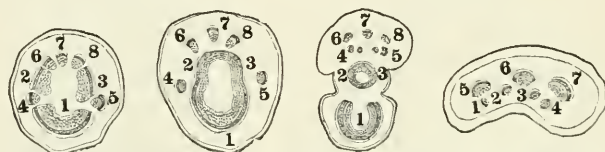
3. ábra. Carpinus betulus : a levélnyalábok kialakulása.
