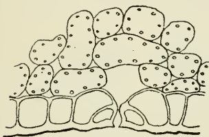
1. ábra. Carpinus betulus lomblevelén lévő levegőnyílás keresztmetszete.
