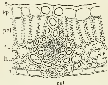
7. ábra. A Carpinus betulus kupacsának keresztmetszete. 450/1. c. = kutikula, ép. = epidermis, pal. = palisádparenchima, scl. = sclerenchima hüvely, f. = farész, h = háncsrész.
