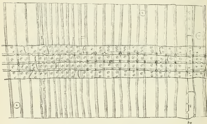
4. rajz. A Biota orientalis fájának radialis metszete. éh: évgűrű határ, hp: hosszparenchyma. 300-szor nagyítva.
