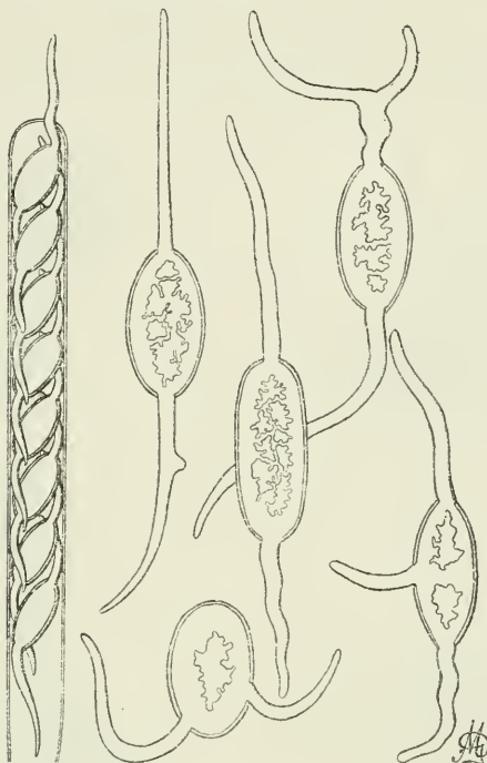
3. kép. A Morchella intermedia Boud. spórái, melyek már az ascusban csiráznak. A kép bal oldalán egy ascus felső része, benne a csirázó spórák, 400-szorosan nagyítva. Az ascustól jobbra öt csirázó spóra, 800-szorosan nagyítva. (Eredeti rajz.)
