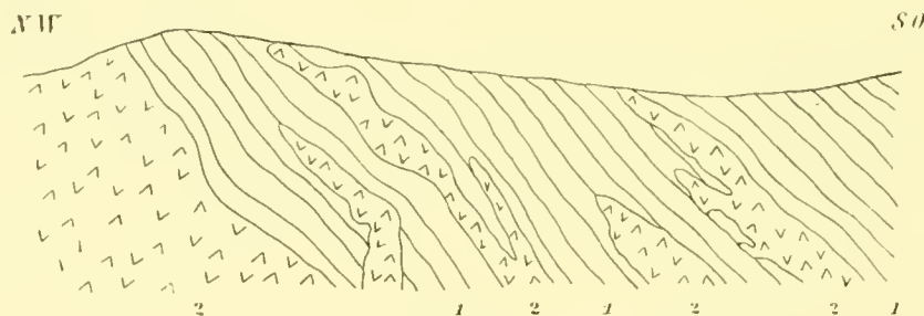
Granitapophysen und Gänge (2) im Gneis (1) bei Bahú.
