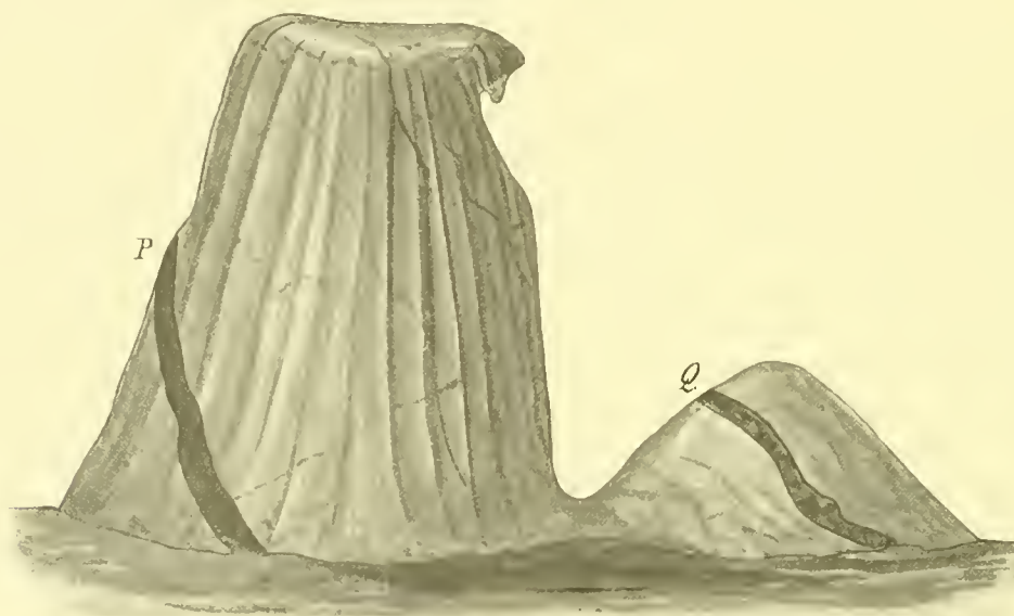
Granit-Erosionskegel mit Regenfurchen bei Floriano Peixoto.
