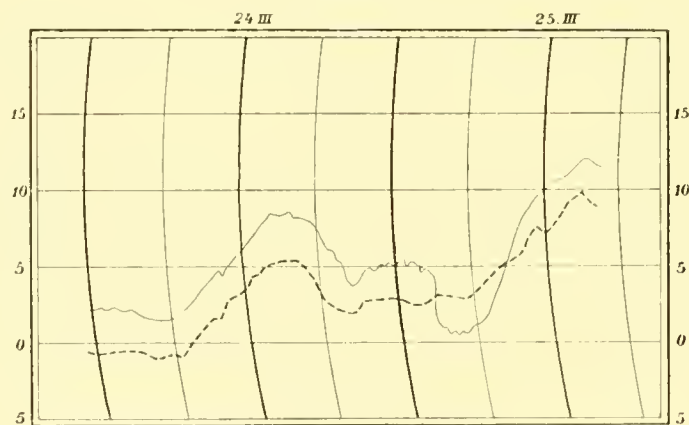
Föhn vom 24.—25. März.
