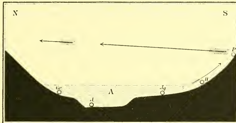
Querprofil durch das Inntal, doppelt überhöht. Luftzirkulation am Morgen des 5. Februar 1904. A stagnierender Bodennebel.
