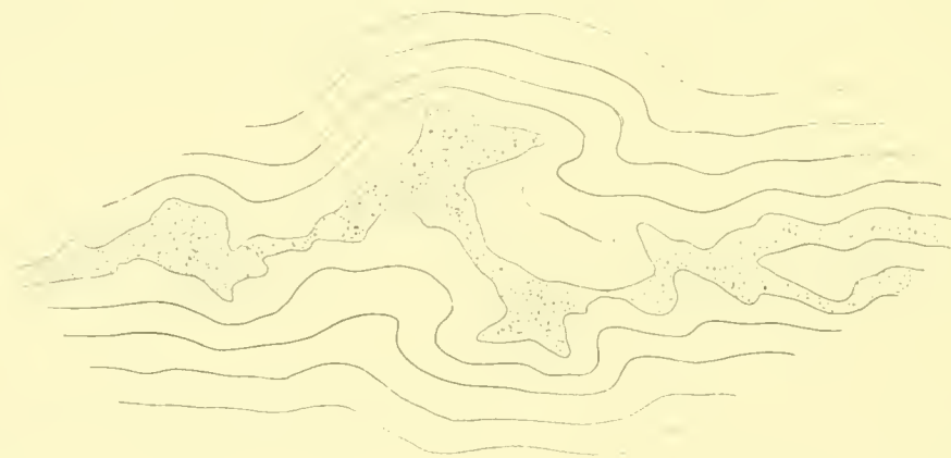
Ein Pressungsnetz im gestauchten Gneis von Aracoyaba. 1 : 12 nat. Gr.
