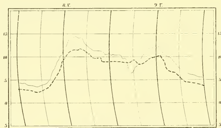
Föhn vom 8.—9. Mai.
