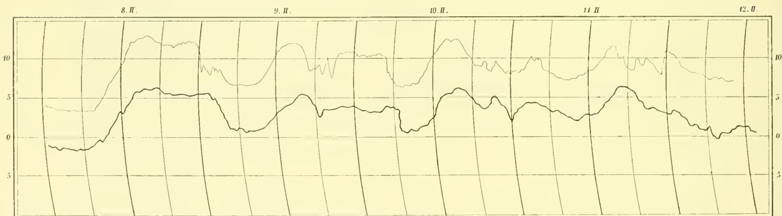
Föhnperiode vom 8.—12. Februar.
