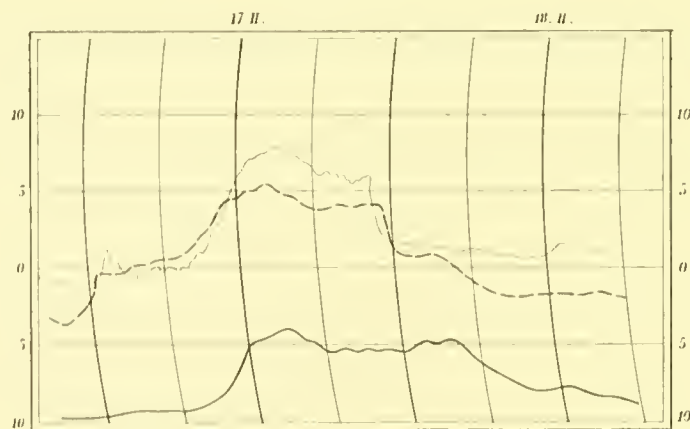
Föhn am 17. Februar.
