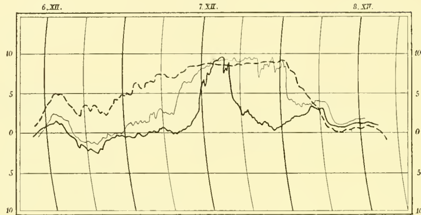
Föhn vom 6.—8. Dezember 1904.
