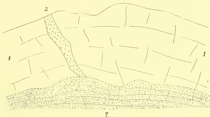
Basische Ausbildung (2) als Tiefenfacies des feldspatreichen porphyrischen Syenites (1). Dieser durchsetzt von einem aplitischen Gang (3).
