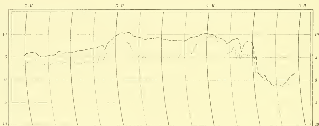
Föhn vom 2.—5. Februar.
