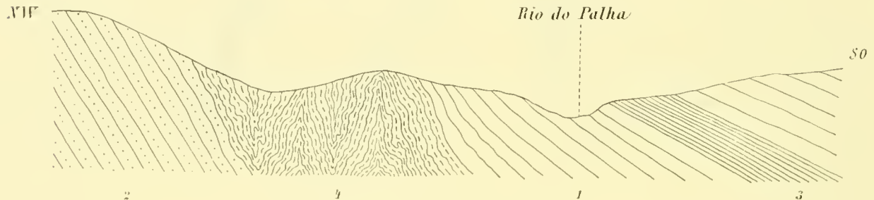
Profil am Ostflusse der Serra Preguiça.
