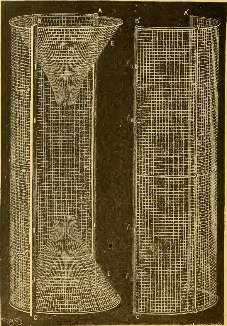
FIG. 8.—Nasa metálica empleada en 1887 y 1888. BC , AD , B'C' y A'D' son las barras de madera y EE son las entradas de la nasa. La reunión de las dos mitades del cilindro se logra por medio de las bisagras f y de pasadores que se introducen en ellas.
