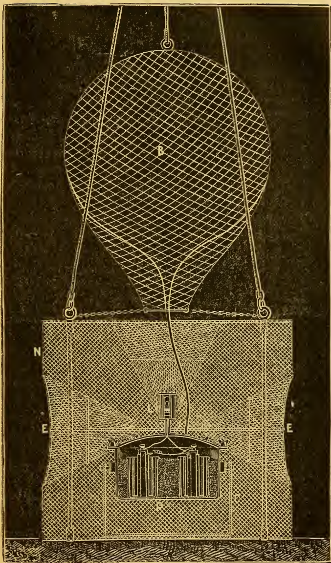
FIG. 12.—Aparato del Dr. Pablo Regnard para iluminar las aguas profundas: N , cuerpo de la nasa; E, E , entradas de la misma; P , pila; L , lámpara; C , suspensión á la Cardan; B , globo compensador de la presión.
