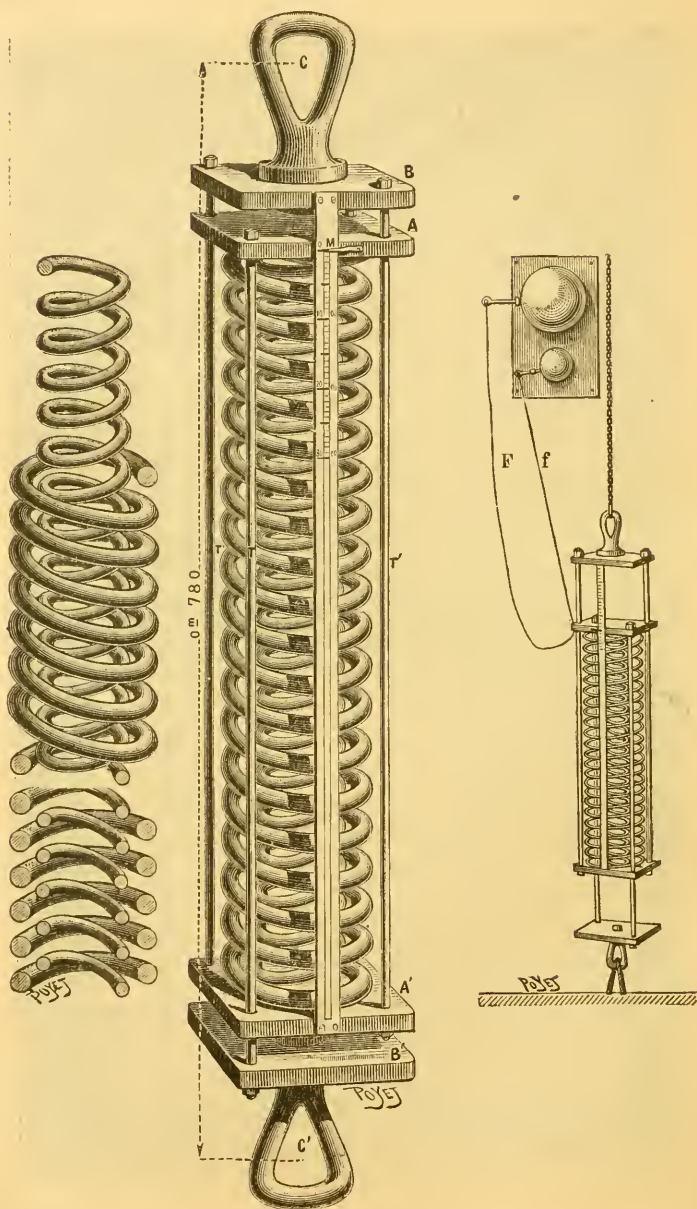
FIGURAS 13, 14 y 15.—Dinamómetro doble de la Hirondelle .
