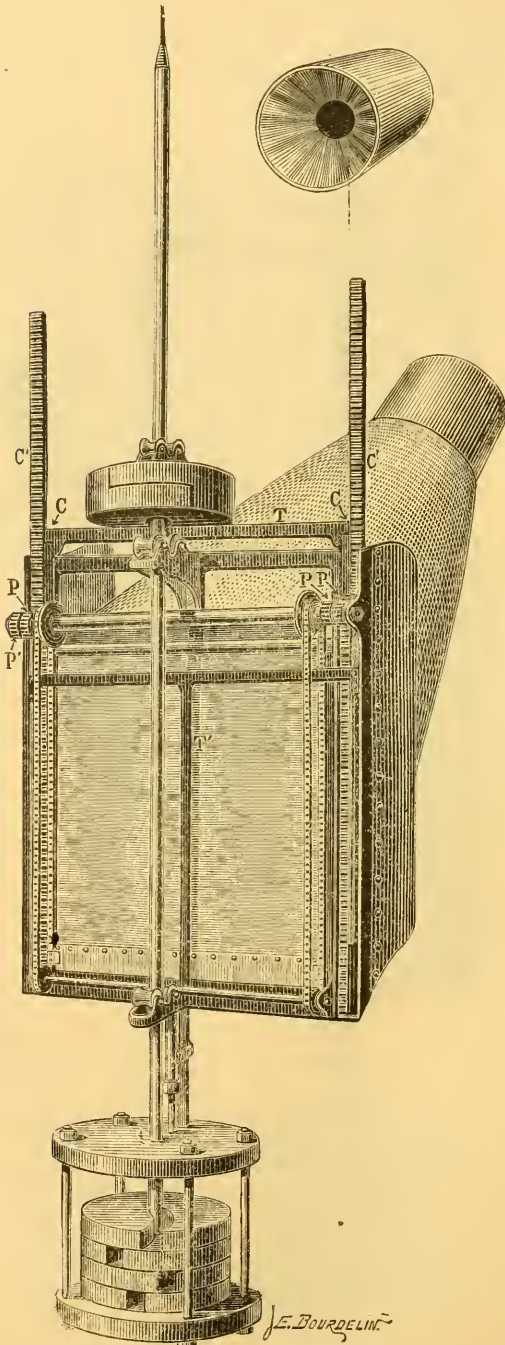
FIG. 7.—El mismo aparato cerrado y subiendo. En la parte superior se representa el frasco de depósito aislado y visto por la cara abierta con el objeto de mostrar el diafragma colocado en su abertura á fin de impedir se escapen los animales capturados.
