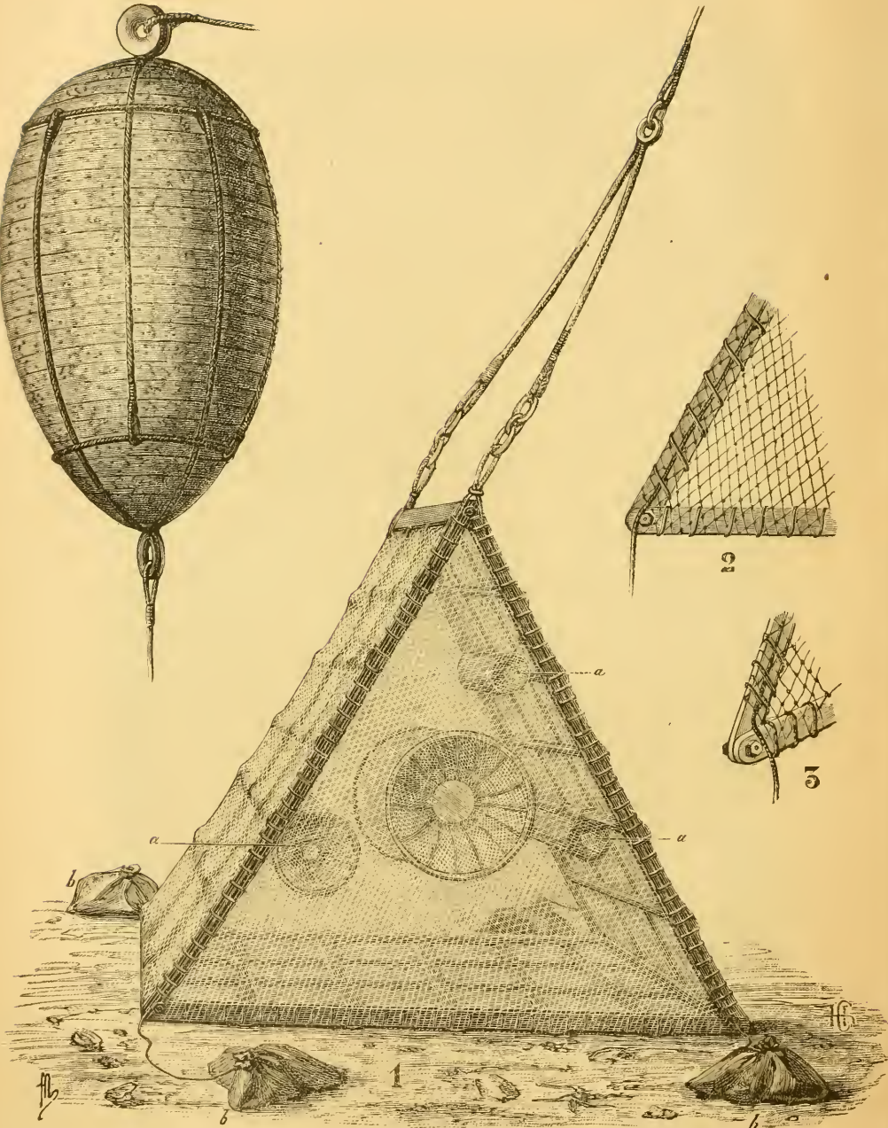
FIG. 9.—Nasa poliédrica construida á bordo de la Hirondelle en 1888.—1. El aparato en su conjunto; a , nasas de tela metálica colocadas en su interior; b , sacos llenos de lastre.—2 y 3. Detalles del aparato para explicar el modo de articulación de las barras de hierro que forman el esqueleto del mismo. Altura total 1,46 m.
