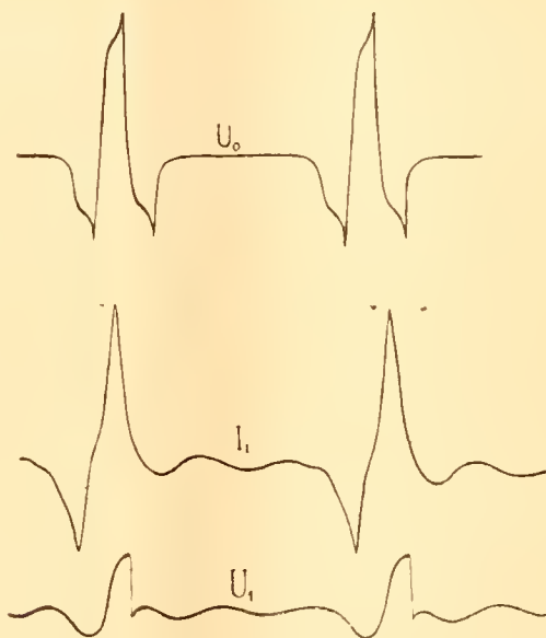
U_0 : tension à vide et courant sur résistance ohmique. I_1 , U_1 : courant et tension sur transformateur chargeant un condensateur relié à un explosif.
