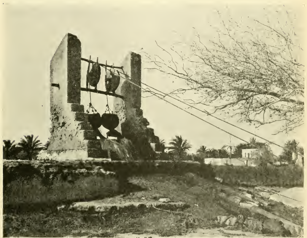
Abb. 3. Wasseraufzug mit zwei Flaschenzügen in der Mencia. Istituto Italiano d'Arti Grafiche, Bergamo.
