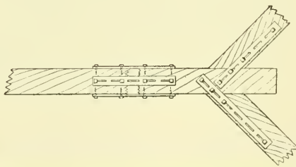
Reparaturschiene für gebrochene Holzteile (Deichsel usw.)
