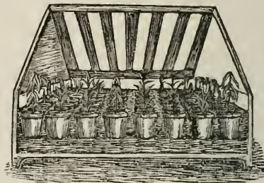
Fig. 5. — Caixão Ward ou estufa de viagem (secção longitudinal).
