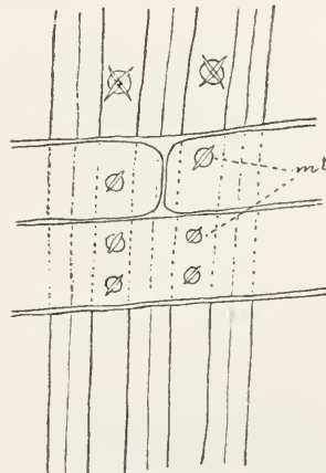
Fig. 3. Radialschnitt durch Spätholz. — mt Markstrahlertüpfel mit spaltenförmigem Porus. Schriff 119 D , Vergr. 400.
