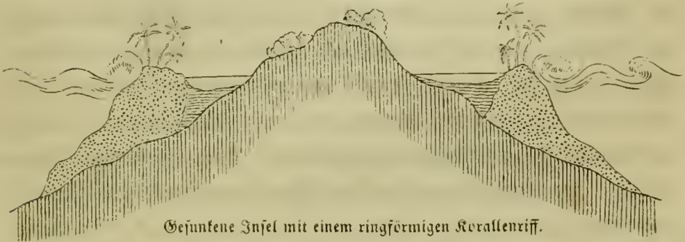
Insel mit einem Kranz von Korallenbänken.
