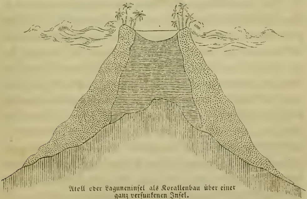
Gesunkene Insel mit einem ringförmigen Korallenriff.
