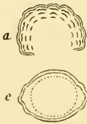
Fig. 1. C. bohemicum .
