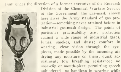
"BURRELL" GAS-MASK.
