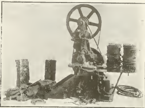
THE MORRIS HEEL-TRIMMER.
