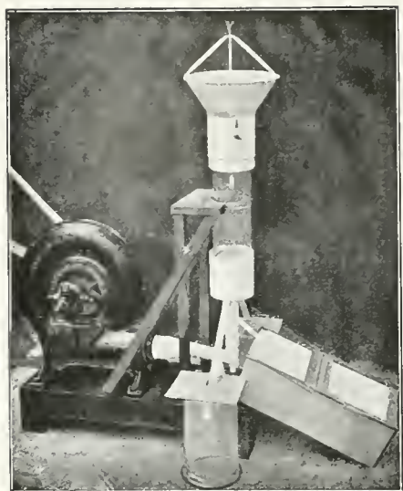
(Foto Collectie Proefst. Vorstenl. tabak). Fig. 36. Zaaduitblazer van het Proefstation te Klaten, (Java).
