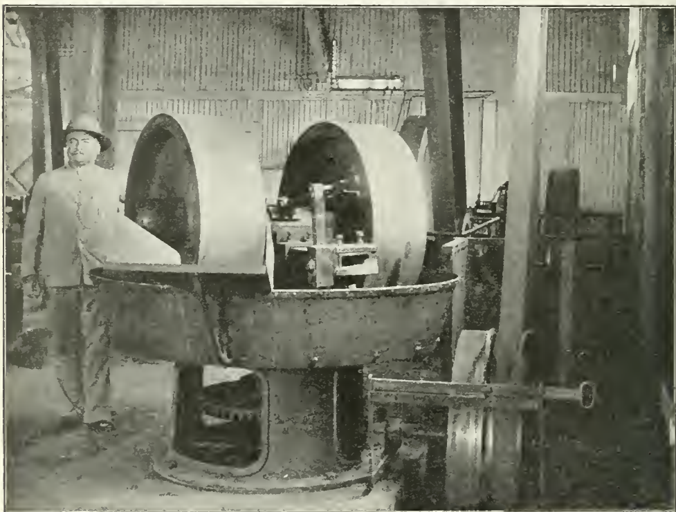
Fig. 108. Kininefabriek te Malabar tot verwerking van versch geoogsten bast.
