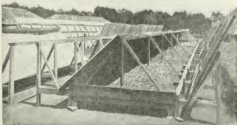
Fig. 103. Droogbakken met losse zinken daken.
