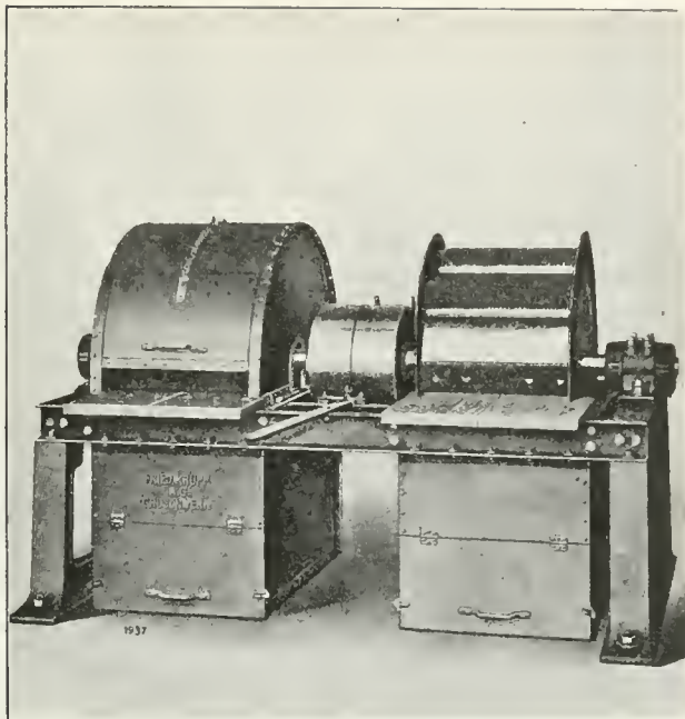
Fig. 169. Borstelmachines.
