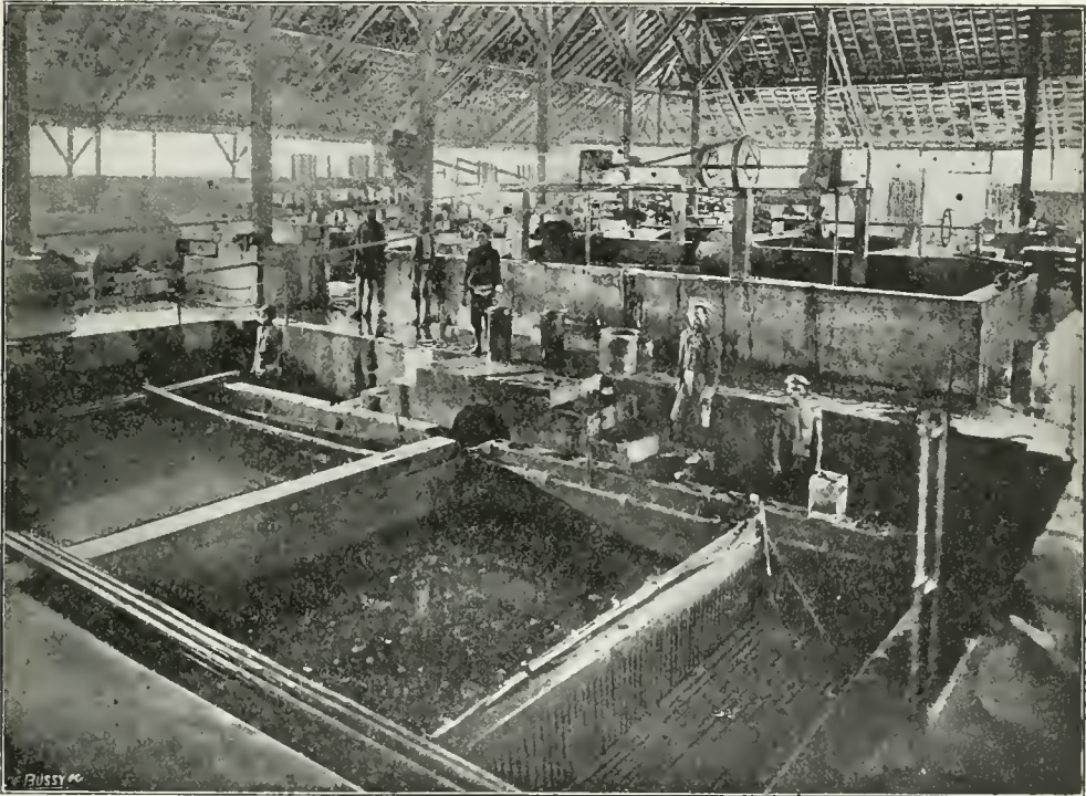
Fig. 195. Doekfilters (voorgrond), zuiveringsbakken voor zwavelzuurbehandeling (achtergrond).
