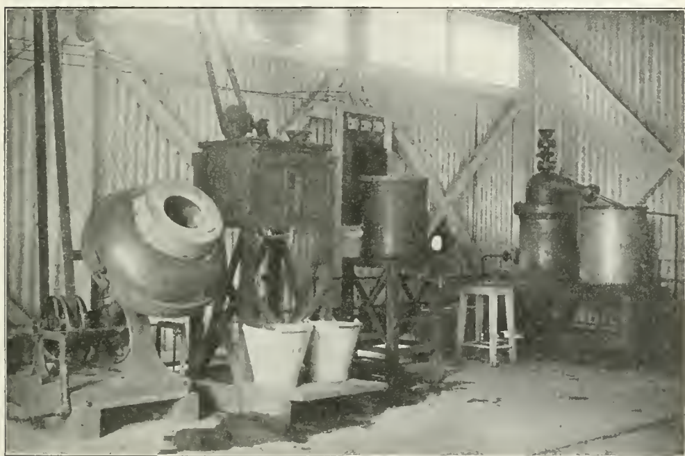
Fig. 100. Proeffabriek te Malabar. — Procédé tot verwerking van versch geoogsten bast.
