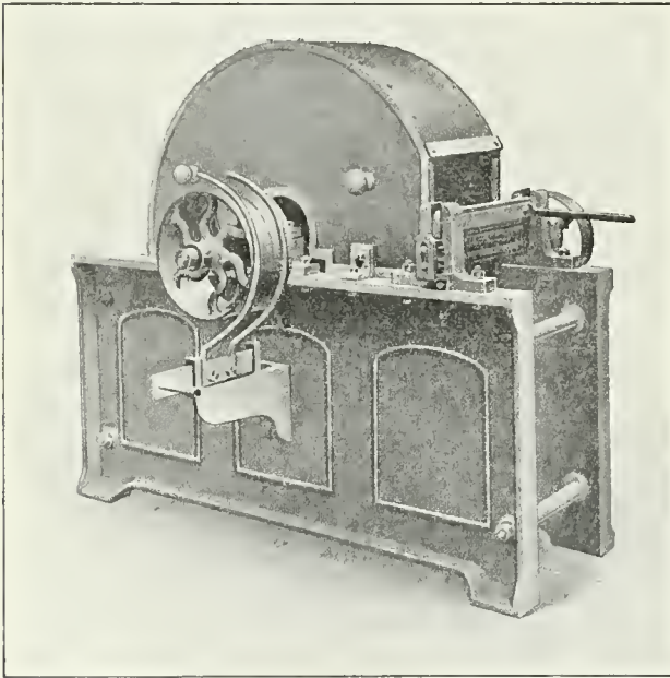
Fig. 162. Ontvezelmaschine.
