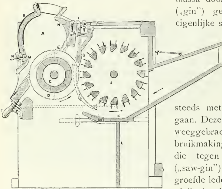
Fig. 149. Dwarse doorsnede door een „sawgin”.
