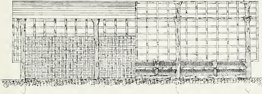
Voor aanzicht. Schaal 1:40.
