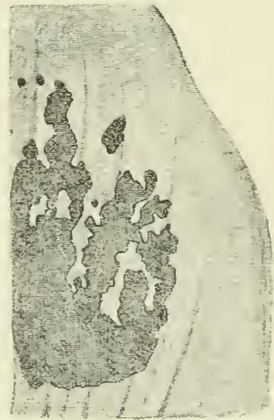
Abbildung 4. Teil einer Zapfenschuppe von Picea excelsa , von der Unterseite zu, mit Spermogonien des Pucciniastrum Padi ( Aecidium strobilinum ). \frac{12}{1}
