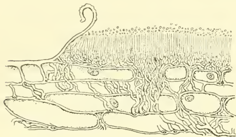
Abbild. 5. Teil eines Längsschnitts durch eine Zapfenschuppe von Picea excelsa mit Spermogonien des Pucciniastrum Padi ( Aecidium strobilinum ) \frac{230}{1}
