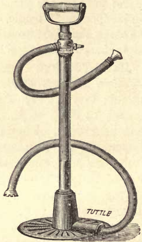
Fig. 125.—EXCELSIOR PUMP.
